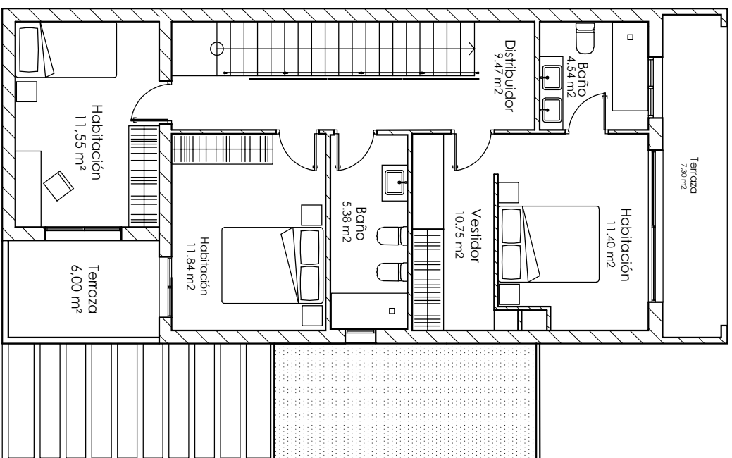
Planta Alta
