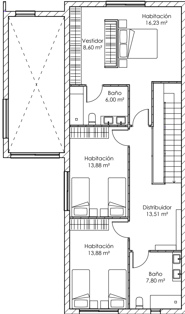
Planta Alta
